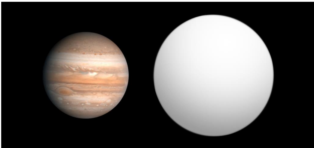
La planète HAT-P-9b ou „Aleph“ (photo : Aldaron, a.k.a. Aldaron/Wikimedia).
